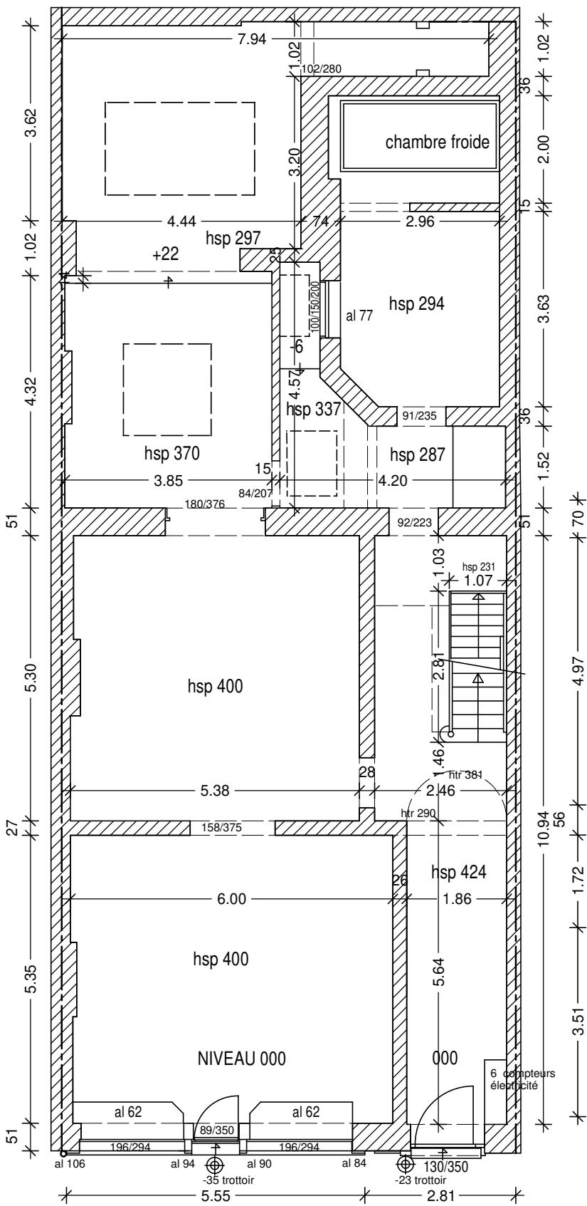
REZ-DE-CHAUSSEE
