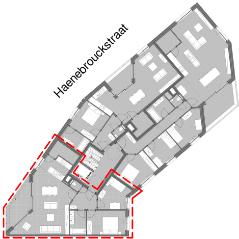
Grondplan
