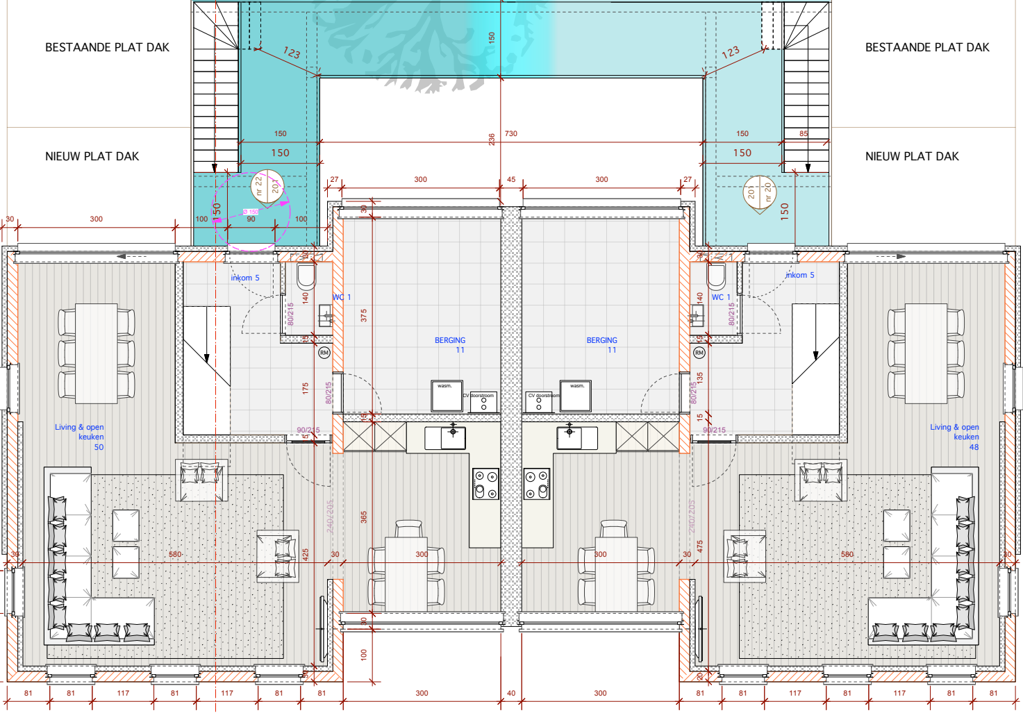
2 de VERDIEPING BRUTO 150 m 2
