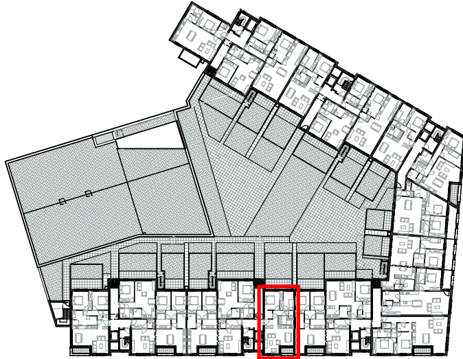
VERDIEPING 2
