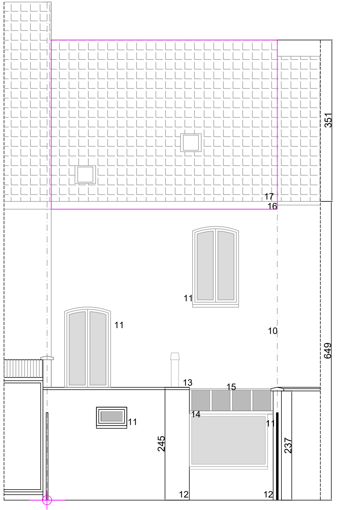
ACHTERGEVEL bestaande toestand - 1/50
