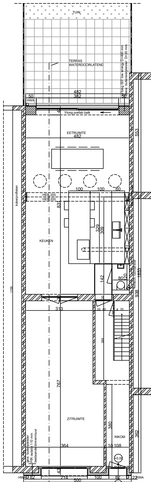
PLAN GELIJKVLOERS nieuwe toestand 1/100
