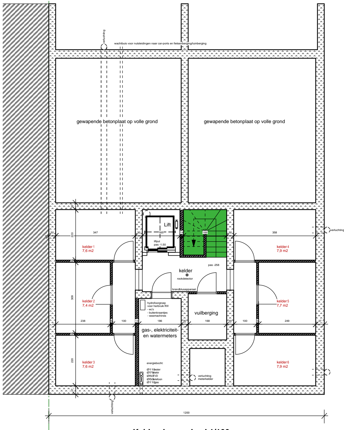
Kelderplan - schaal 1/100
