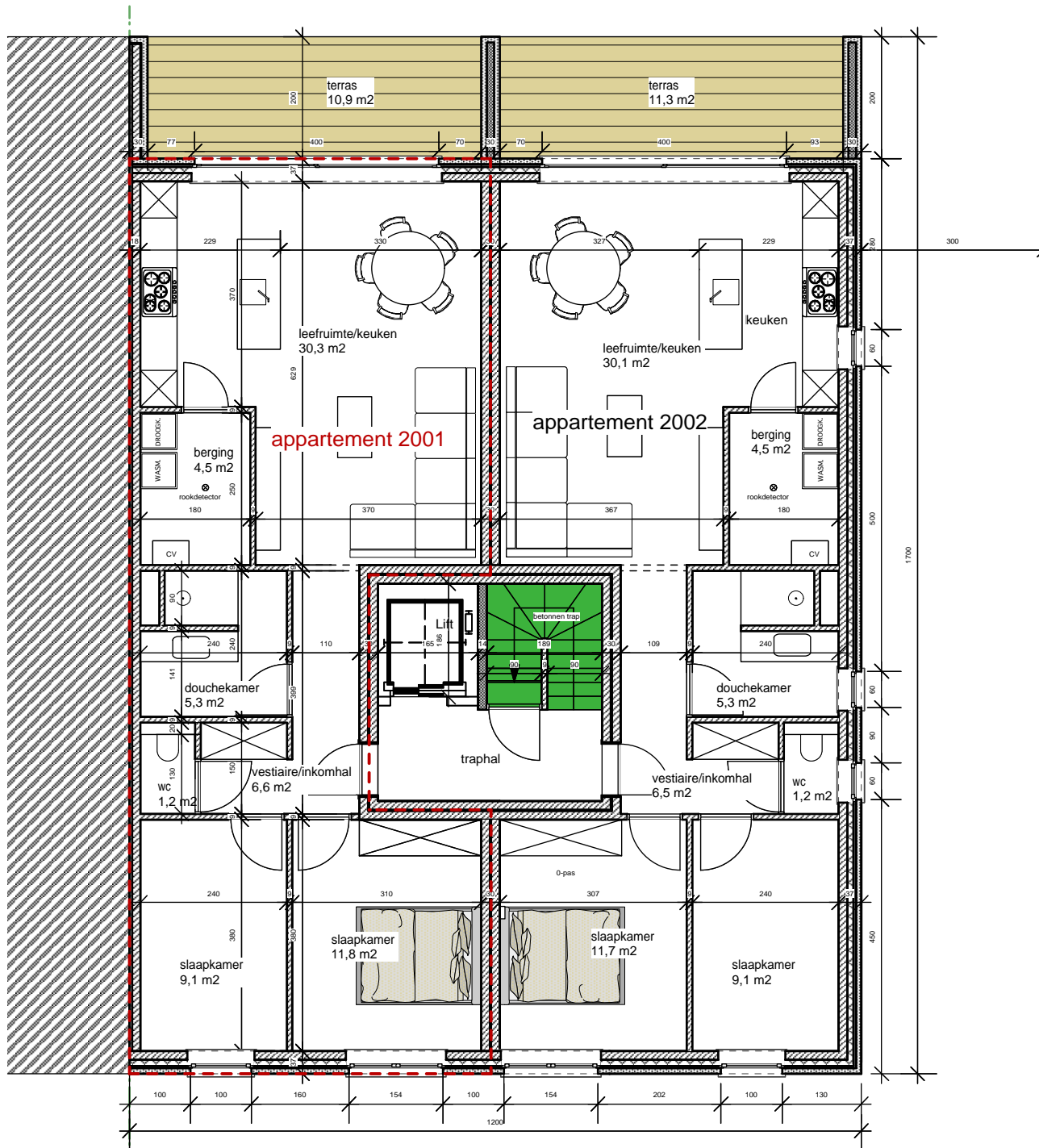
2de verdieping- schaal 1/100
