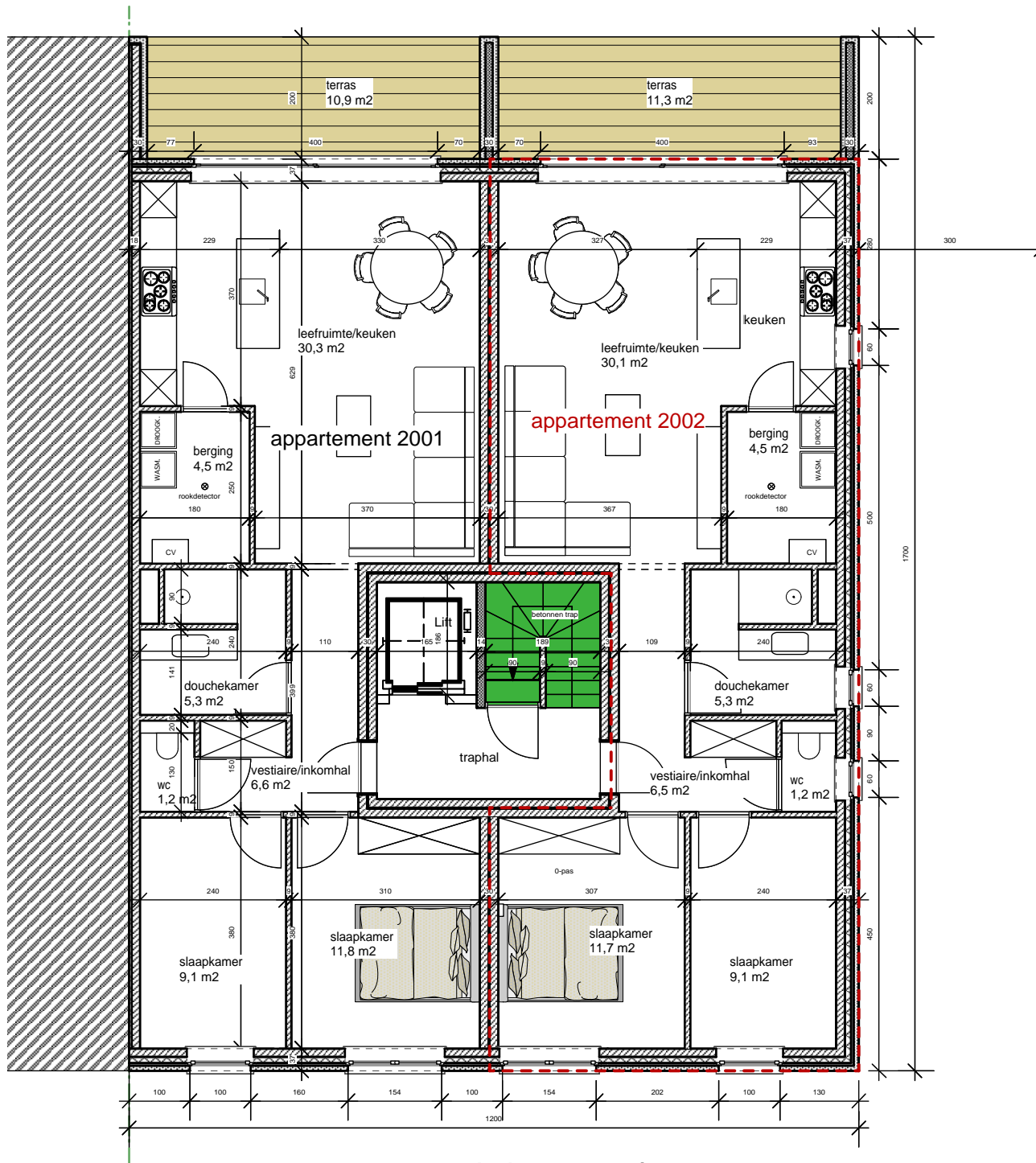
2de verdieping- schaal 1/100
