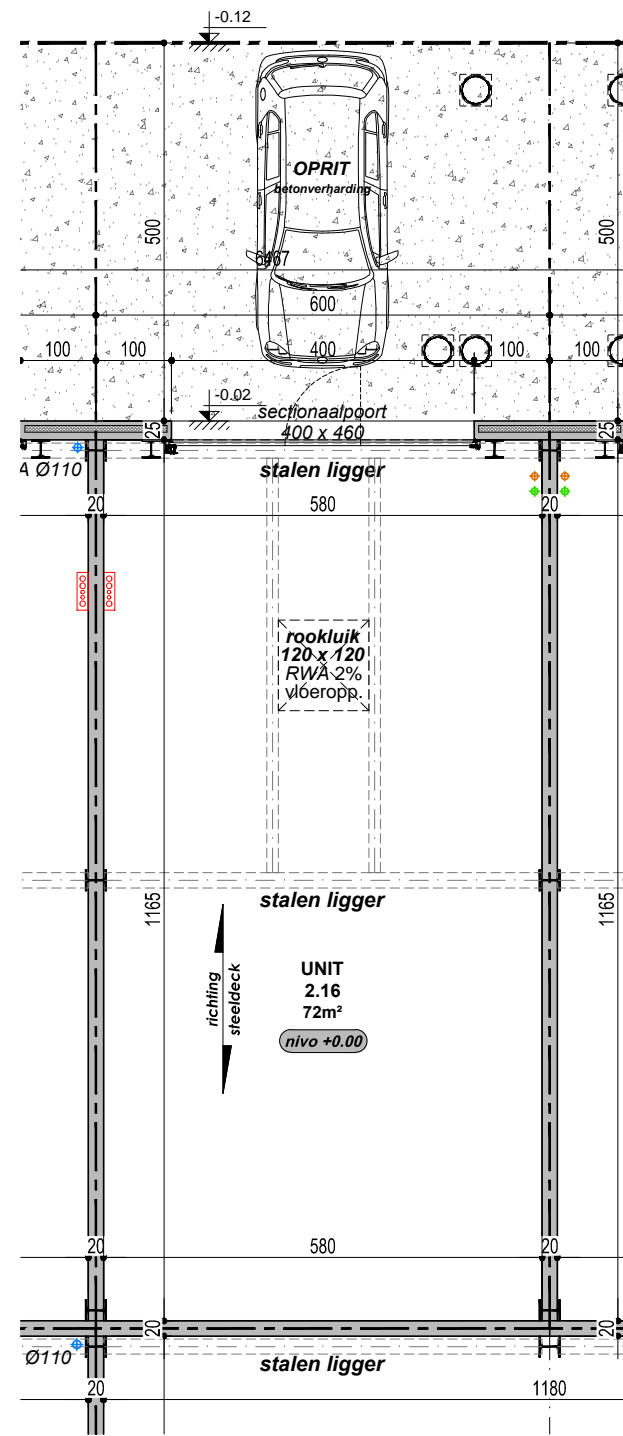
Grondplan
