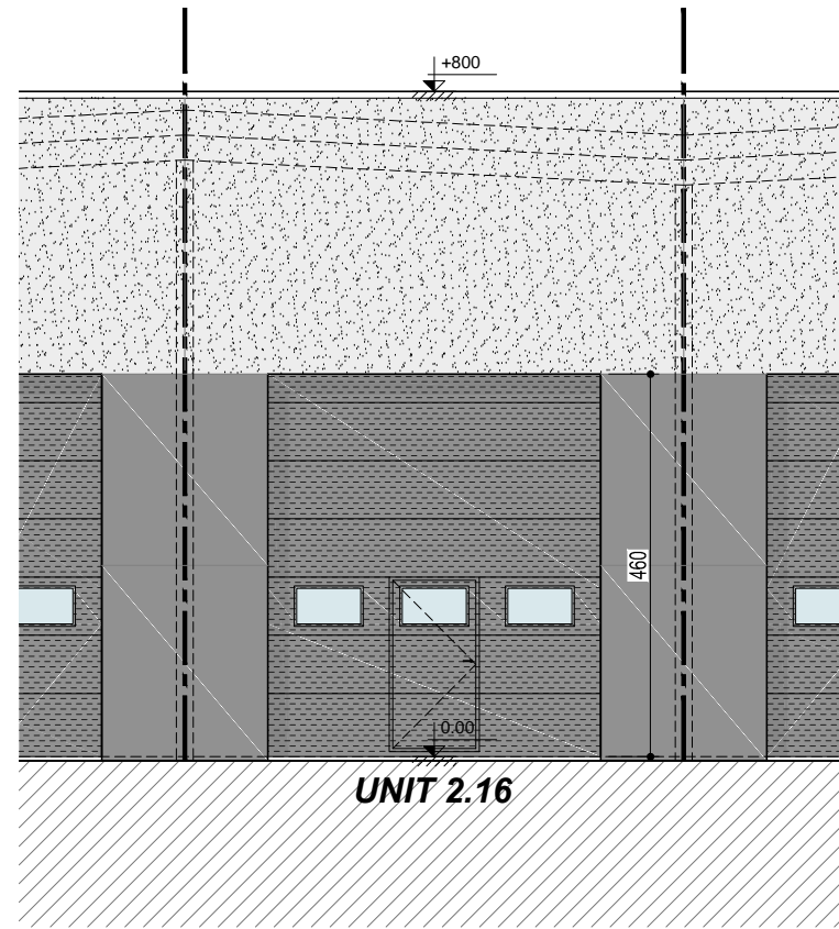
Voorgevel
