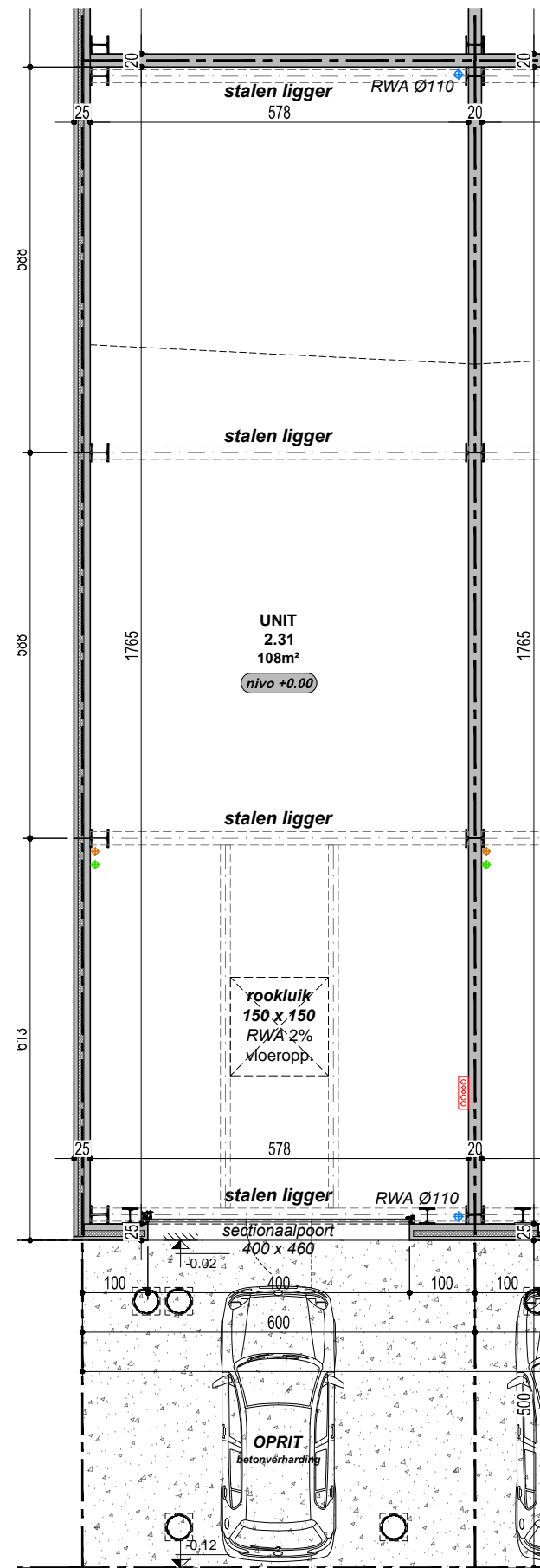
Grondplan
