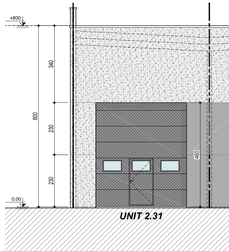
Voorgevel
