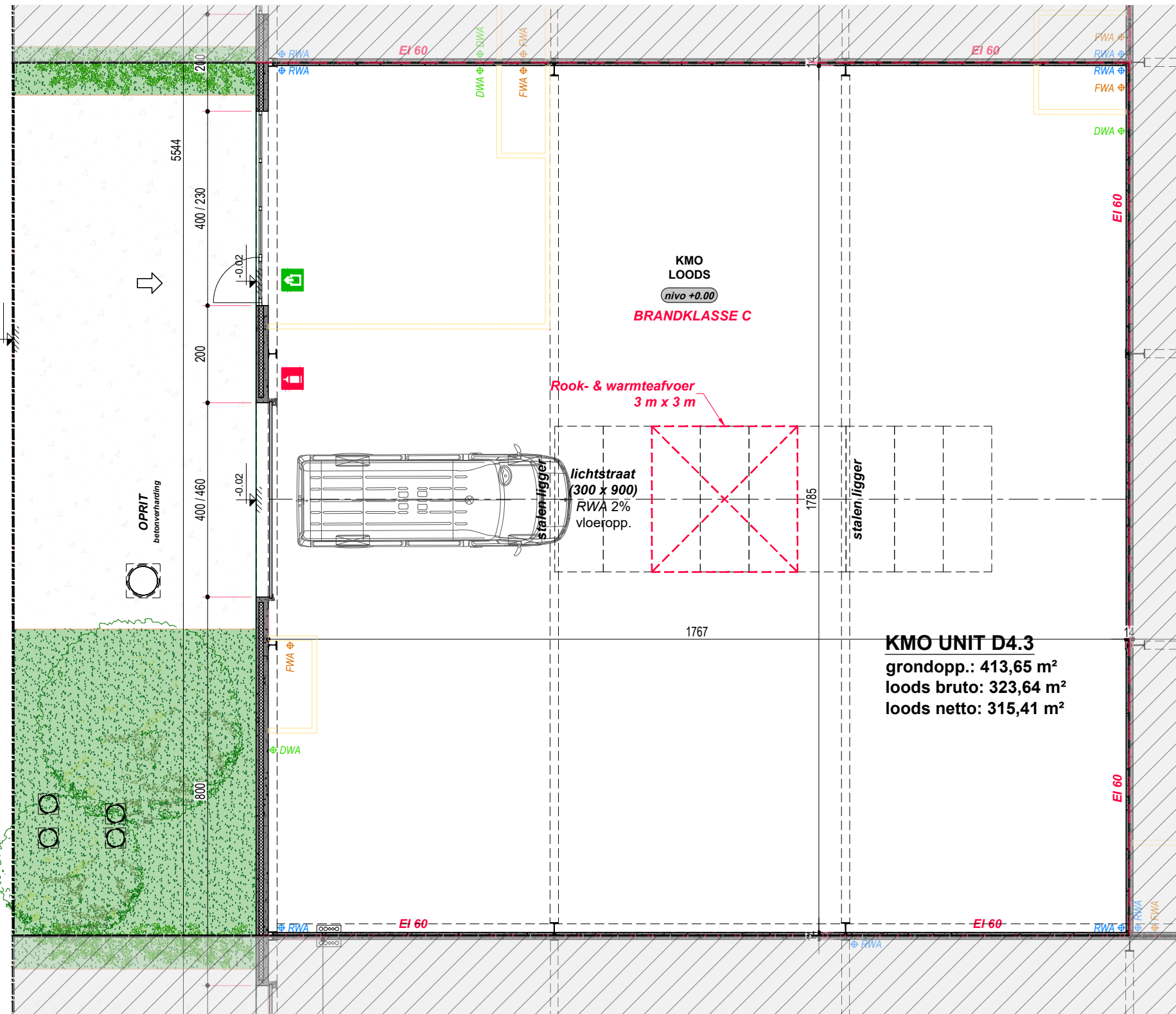
GRONDPLAN
