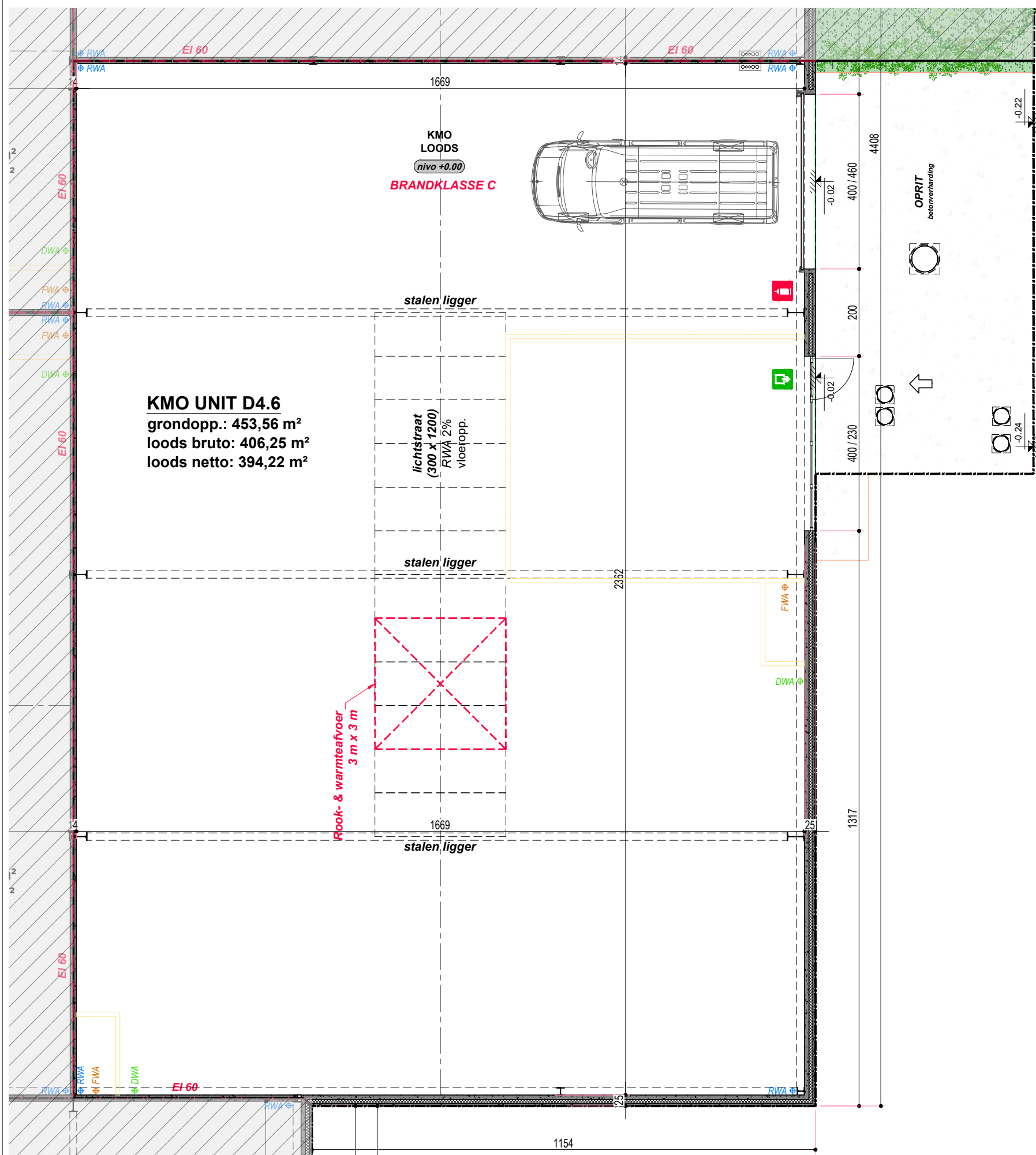
GRONDPLAN
