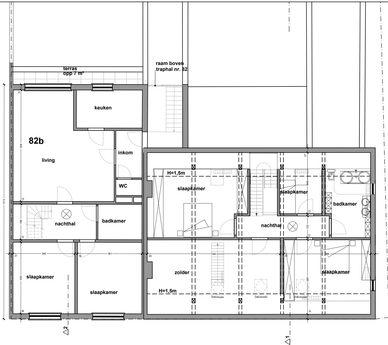
Grondplan 2e verdieping Schaal 1/100
