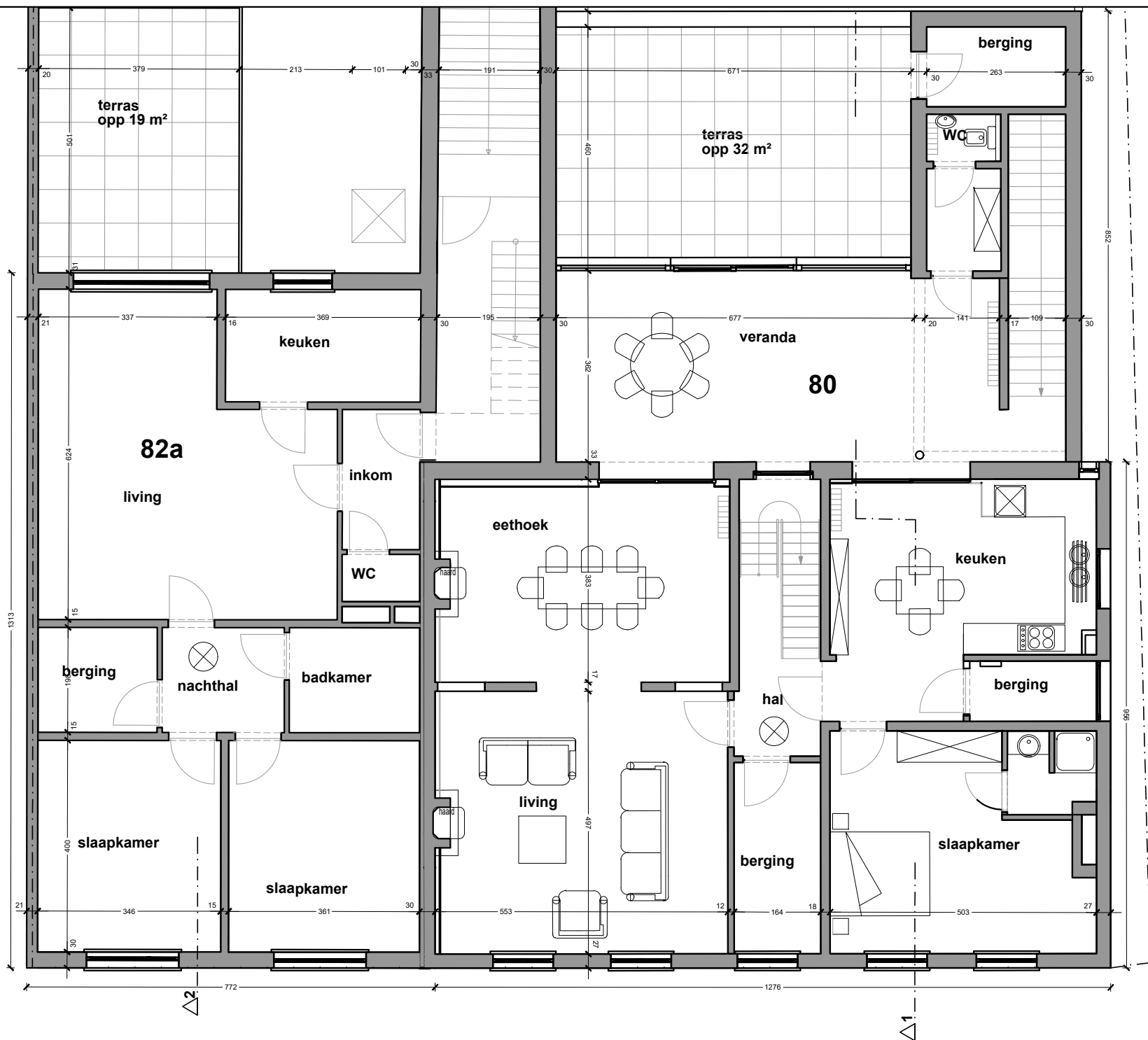
Grondplan 1e verdieping Schaal 1/100
