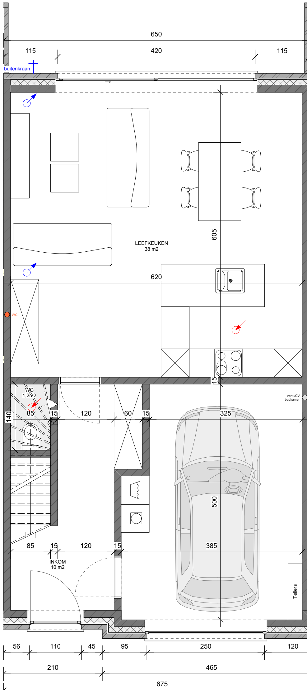
WONING 8: GELIJKVLOERS 78m 2
