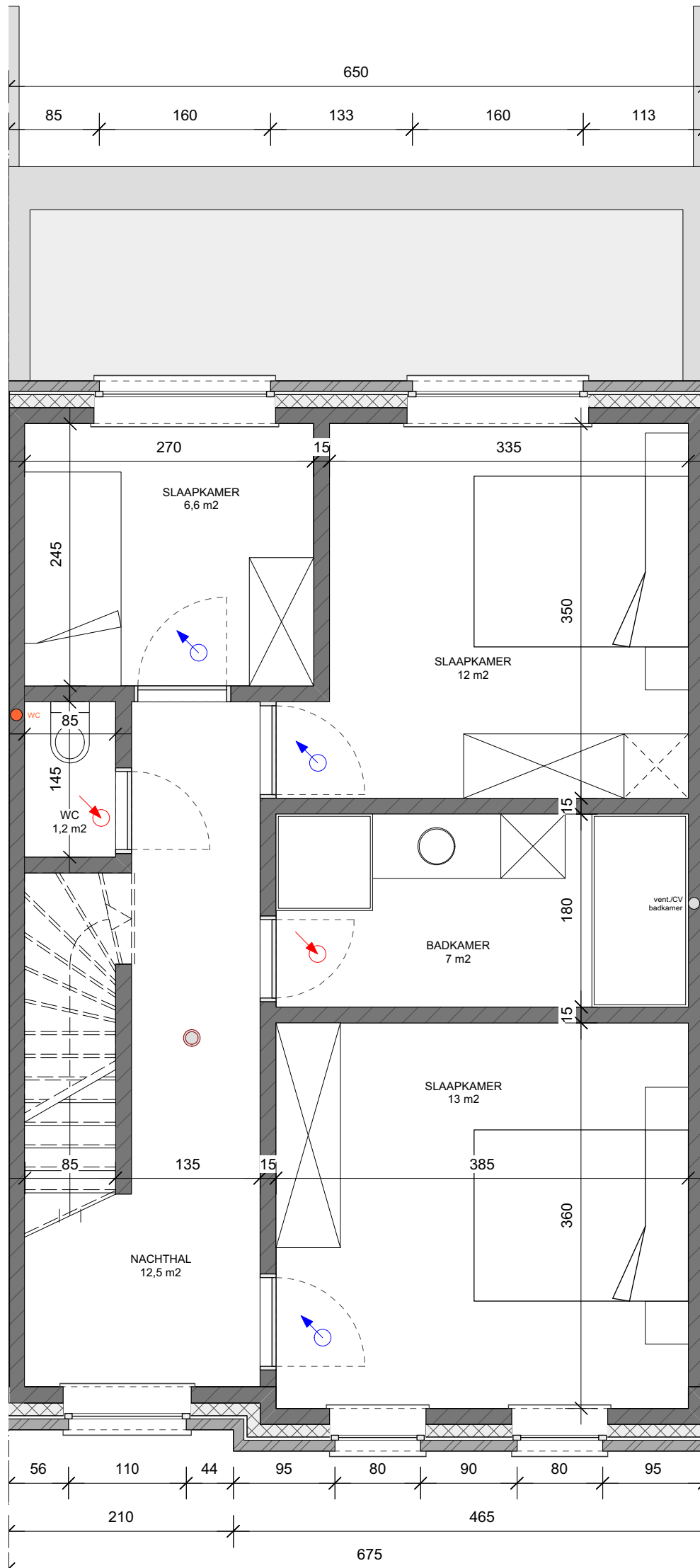
WONING 8: EERSTE VERDIEP 65m 2
