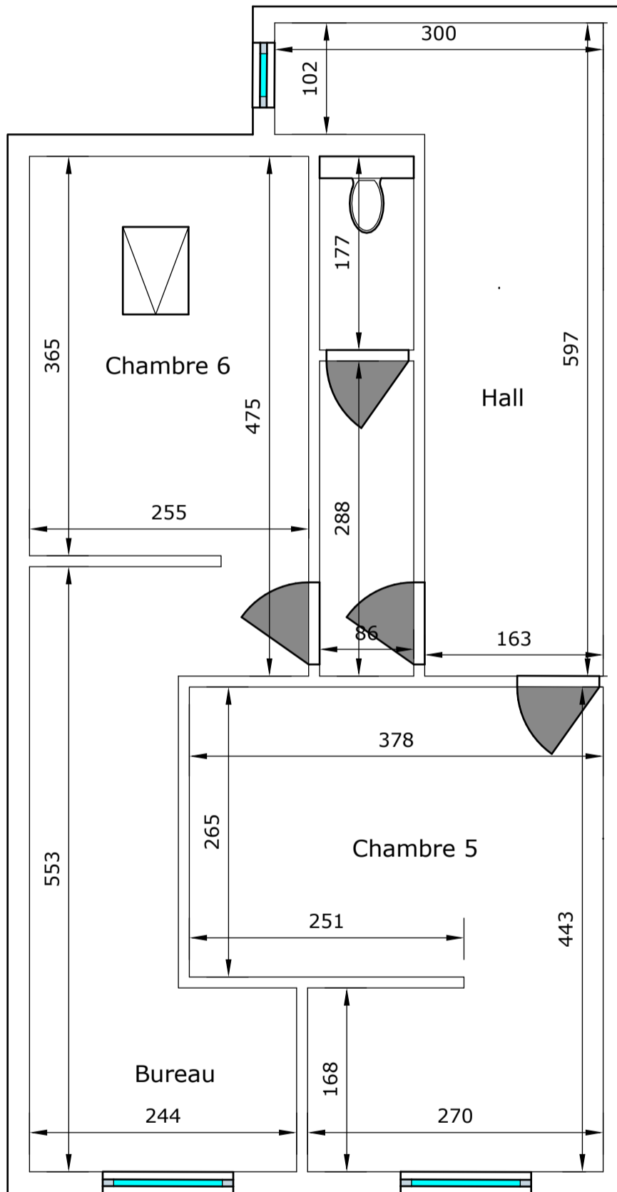
2eme étage
