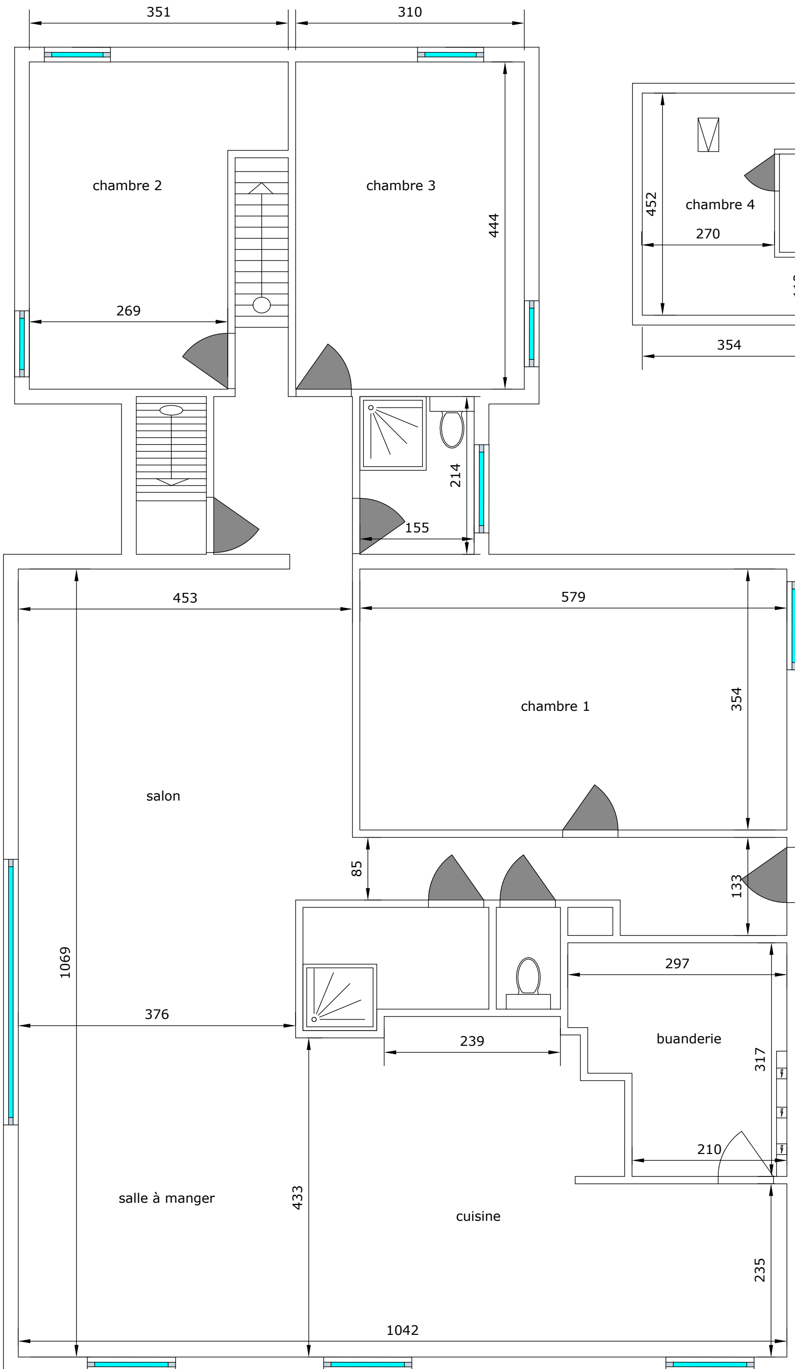
rez-de-chaussée 1:50
