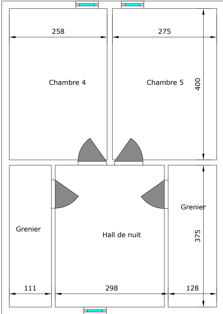
2eme étage 1:50
