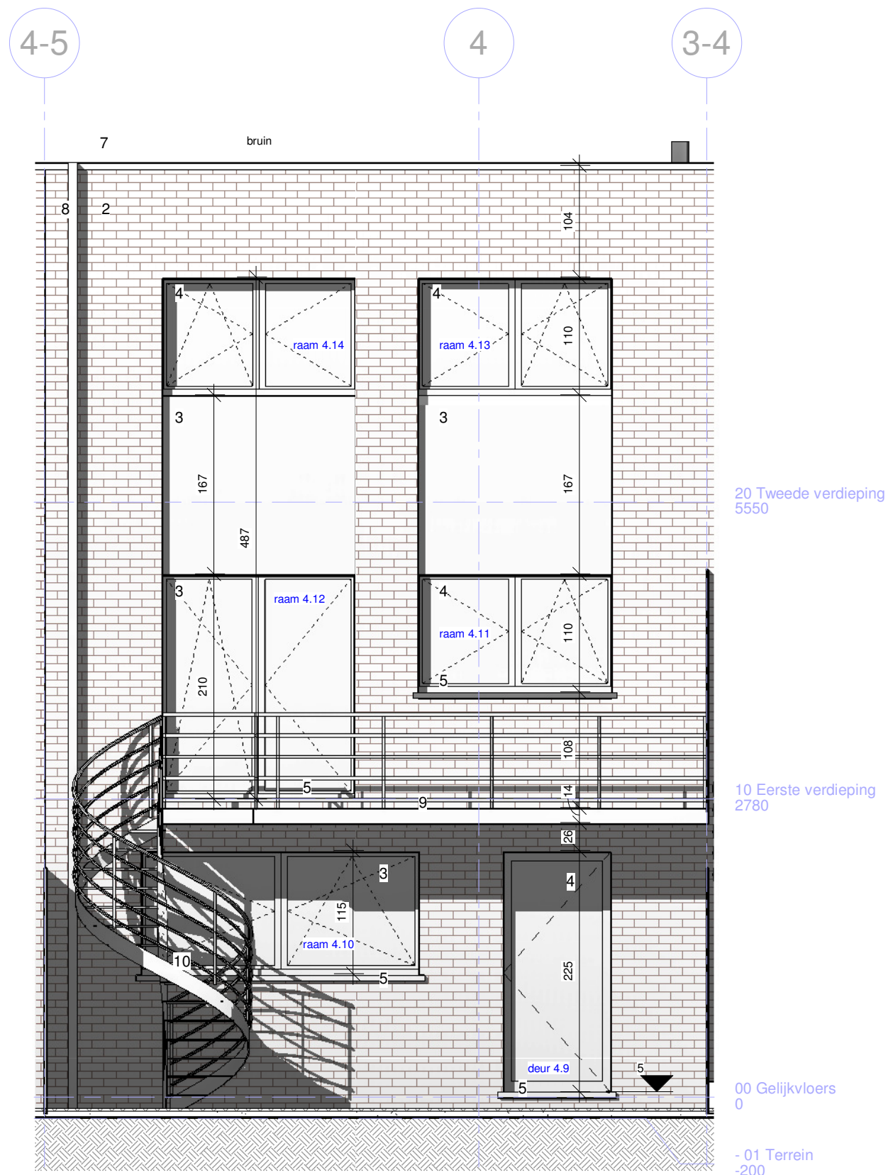
1 Achtergevel woning 4 1 : 50
