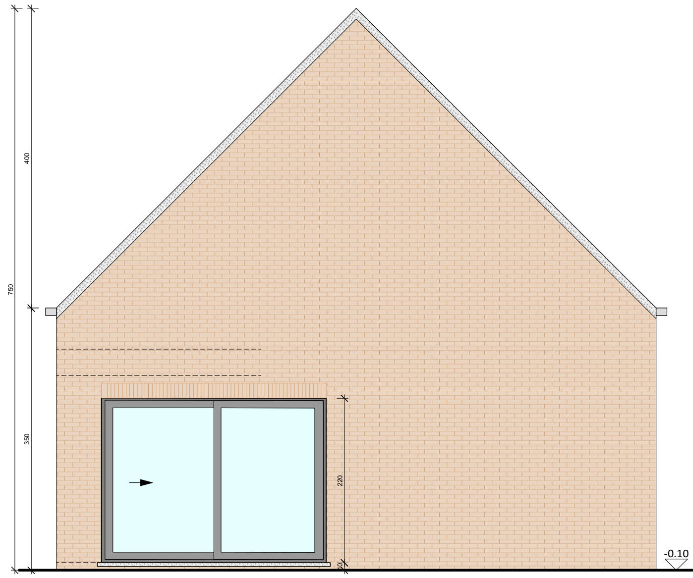
Type 1 Linkerzijgevel
