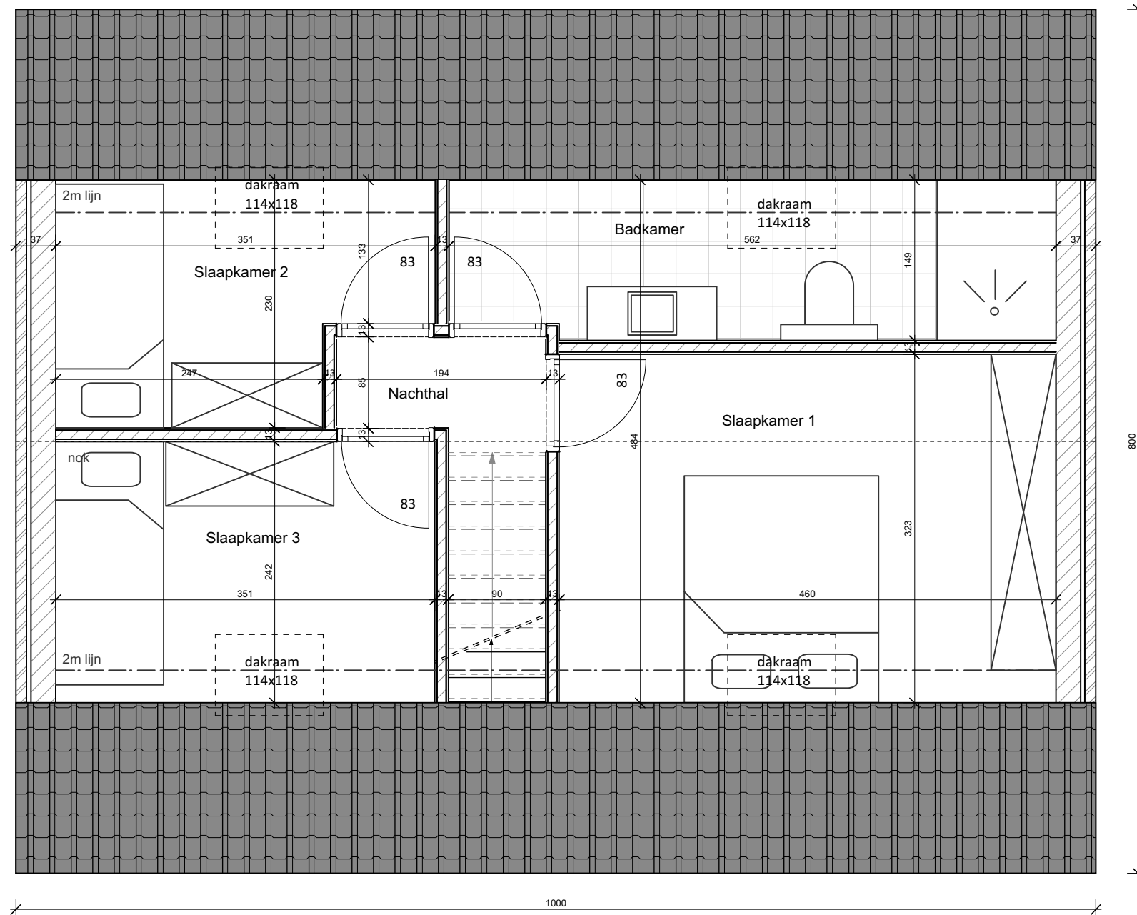
Type 1 Verdiep
