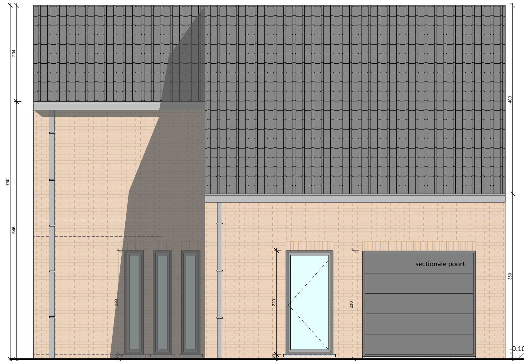
Type 3 Voorgevel
