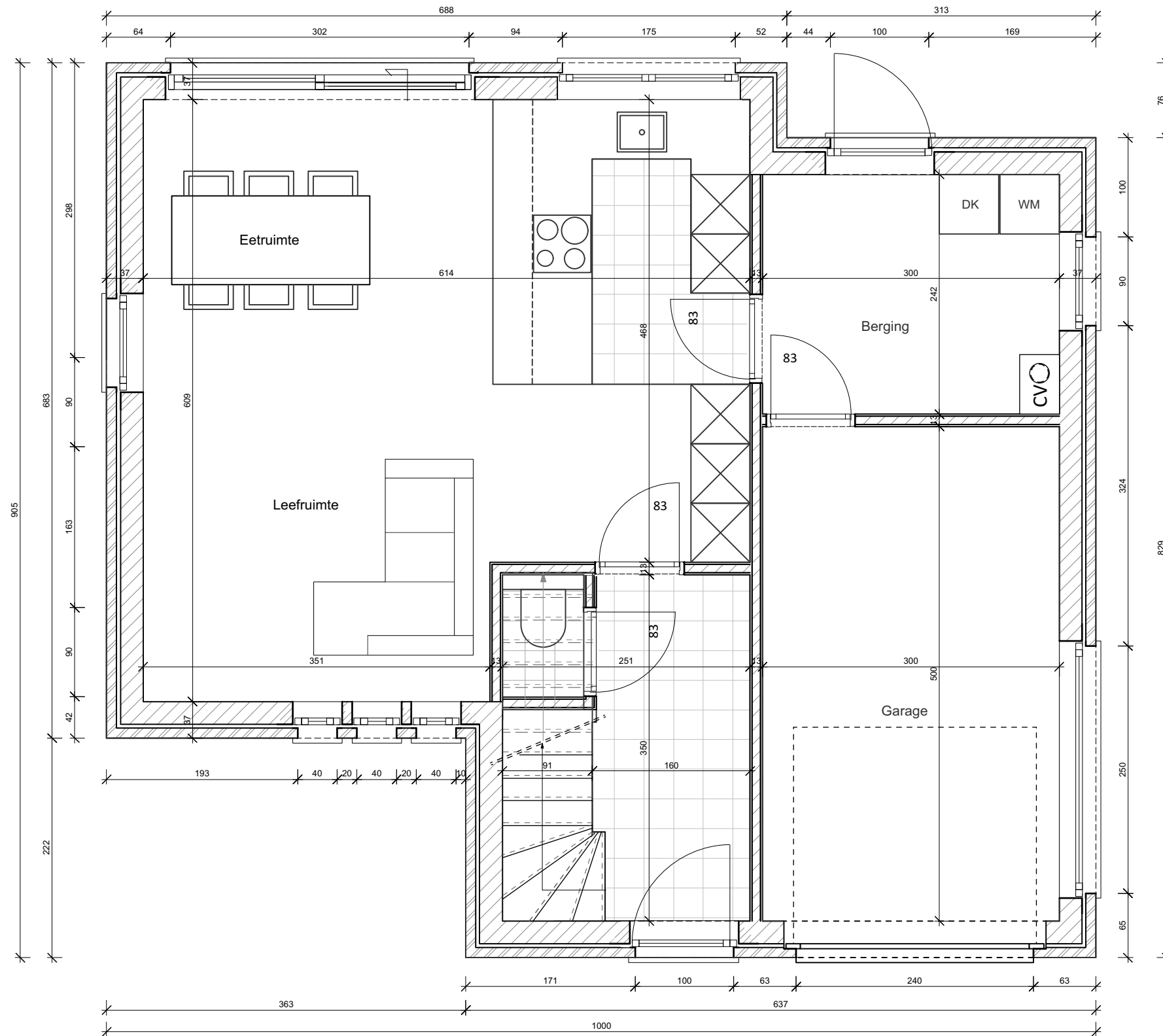
Type 3 Grondplan
