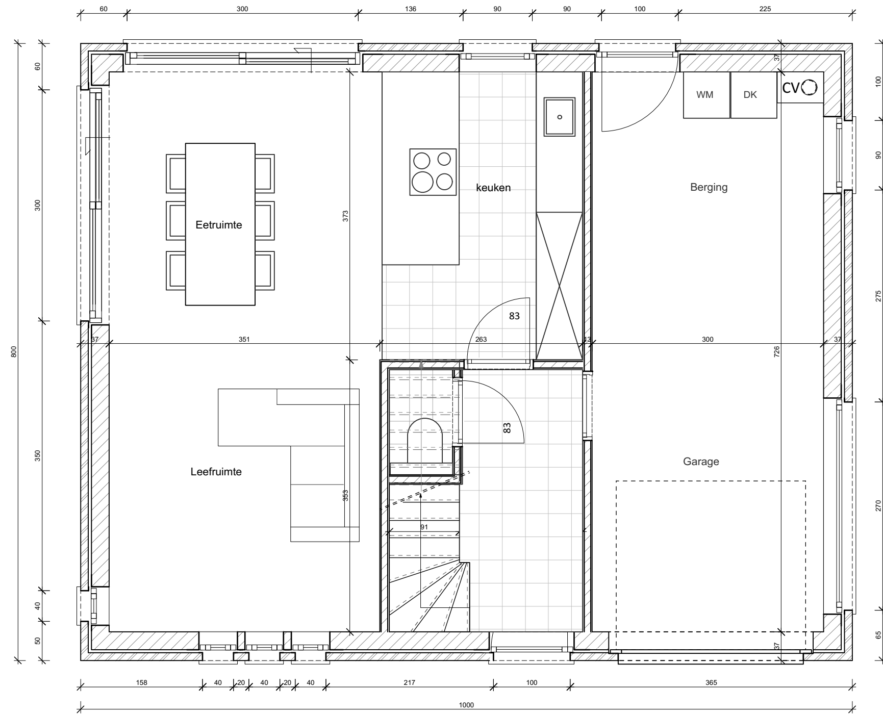
Type 1 Grondplan
