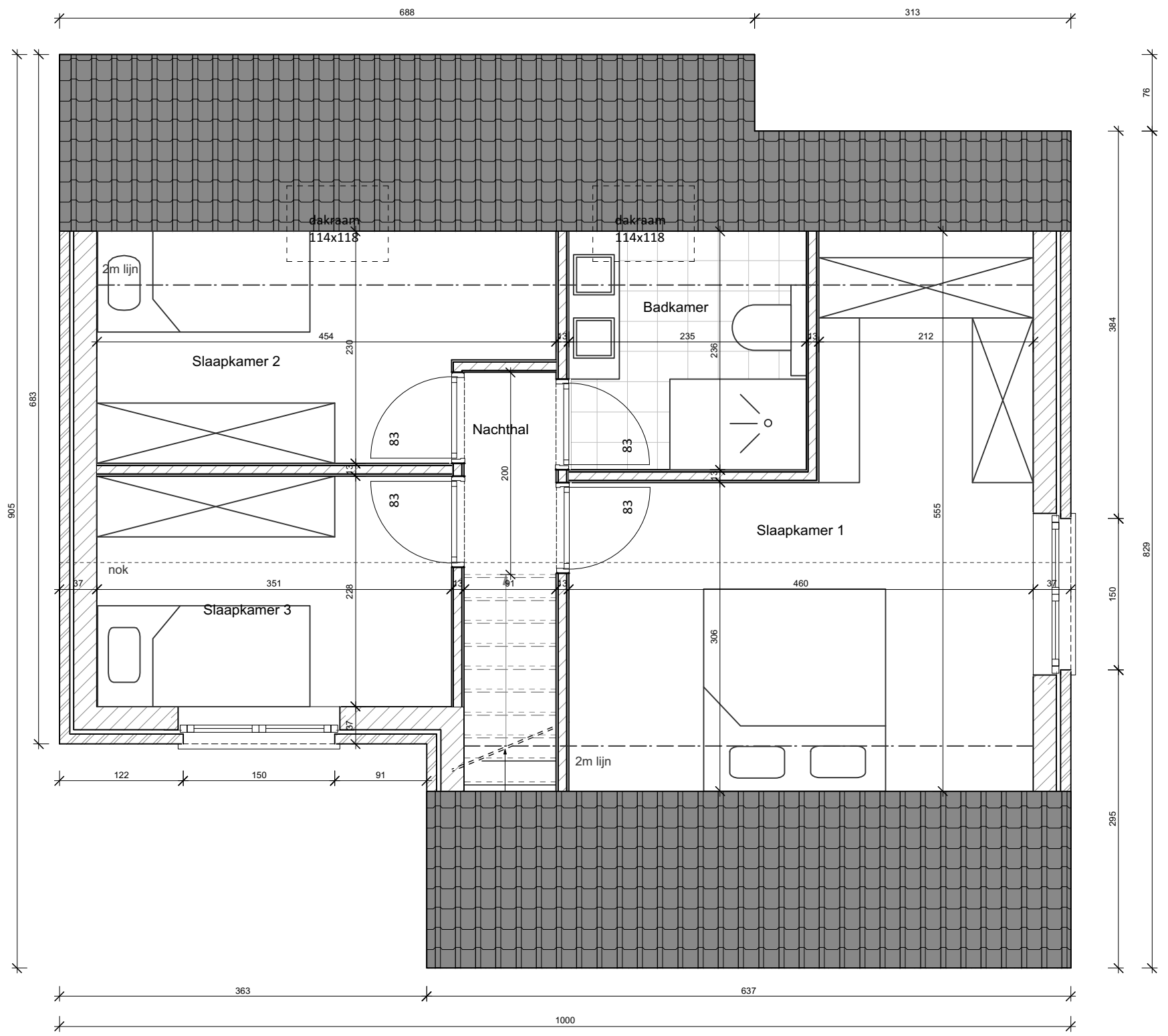
Type 3 Verdiep
