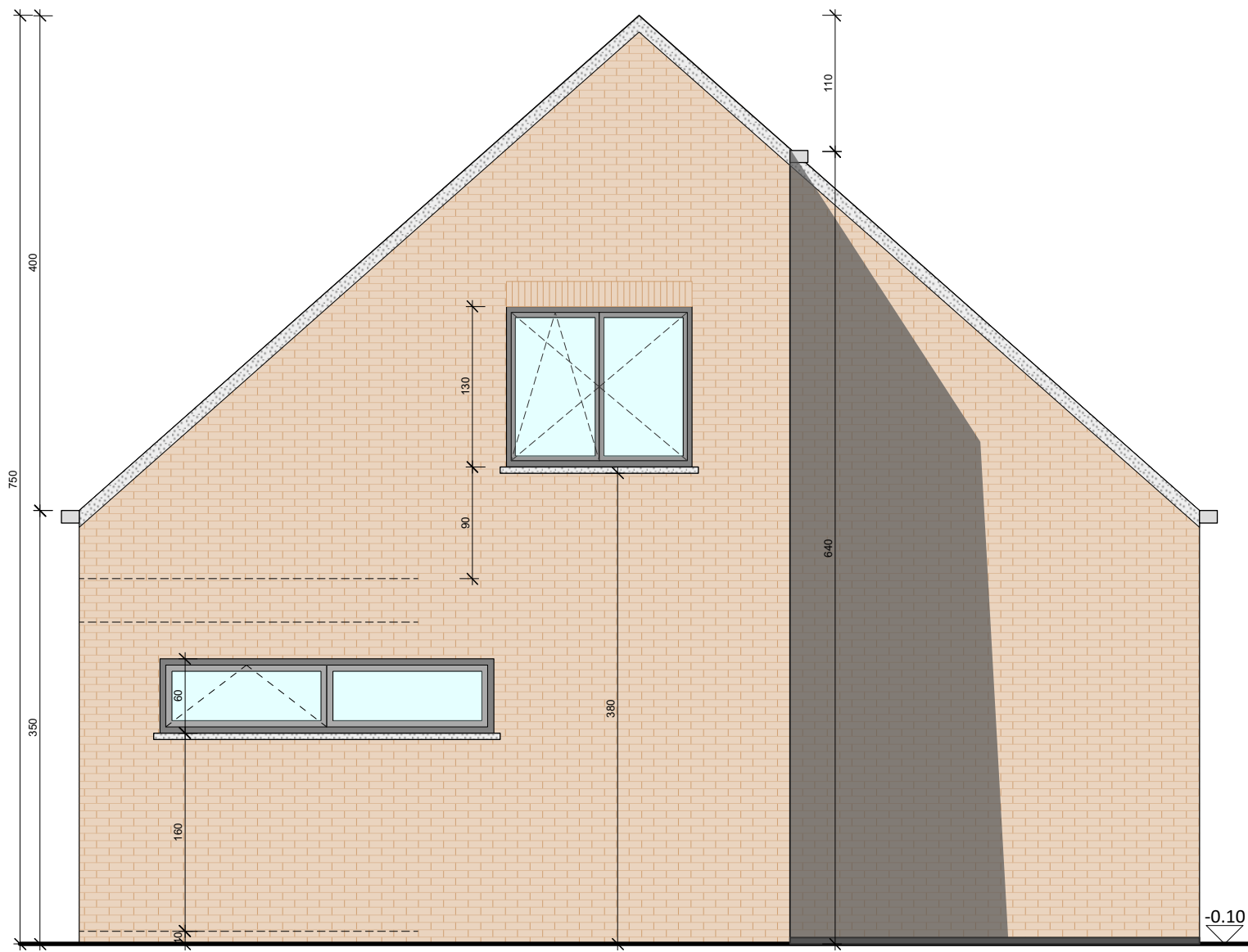
Type 2 Rechterzijgevel
