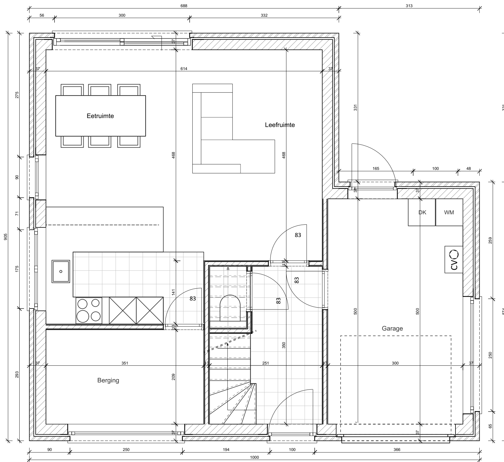
Type 2 Grondplan
