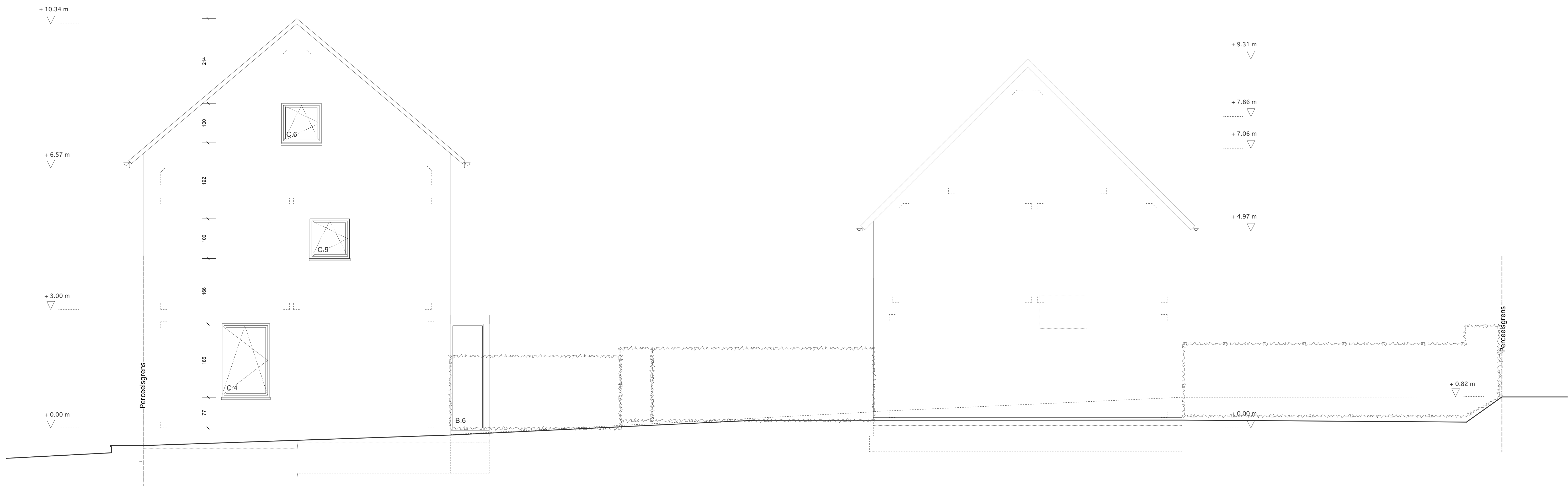
Aanzicht EE' Schaal 1/50
