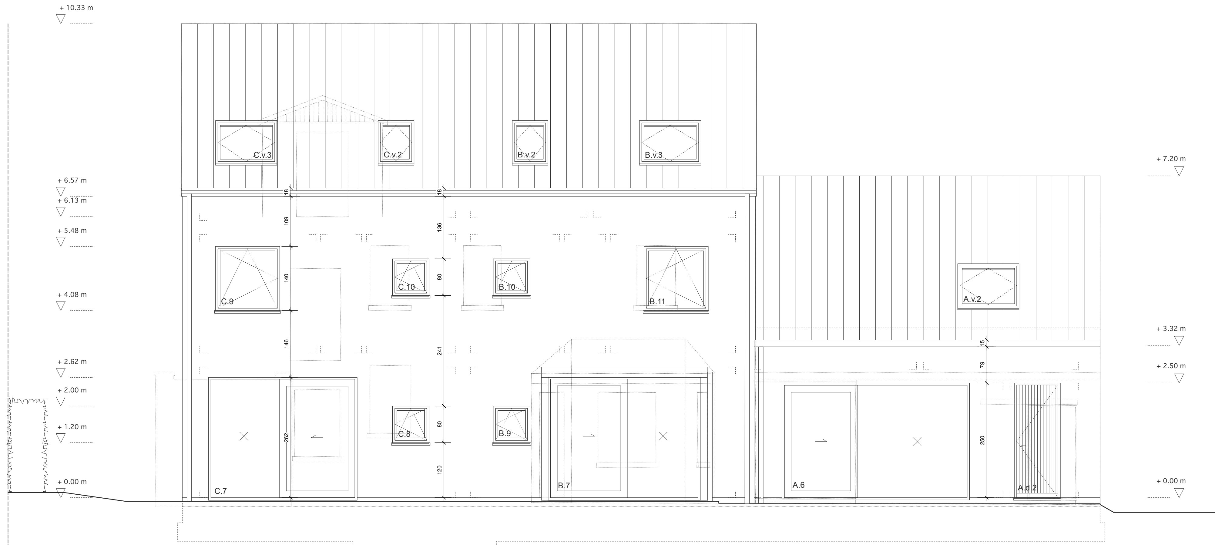
Aanzicht BB' Schaal 1/50
