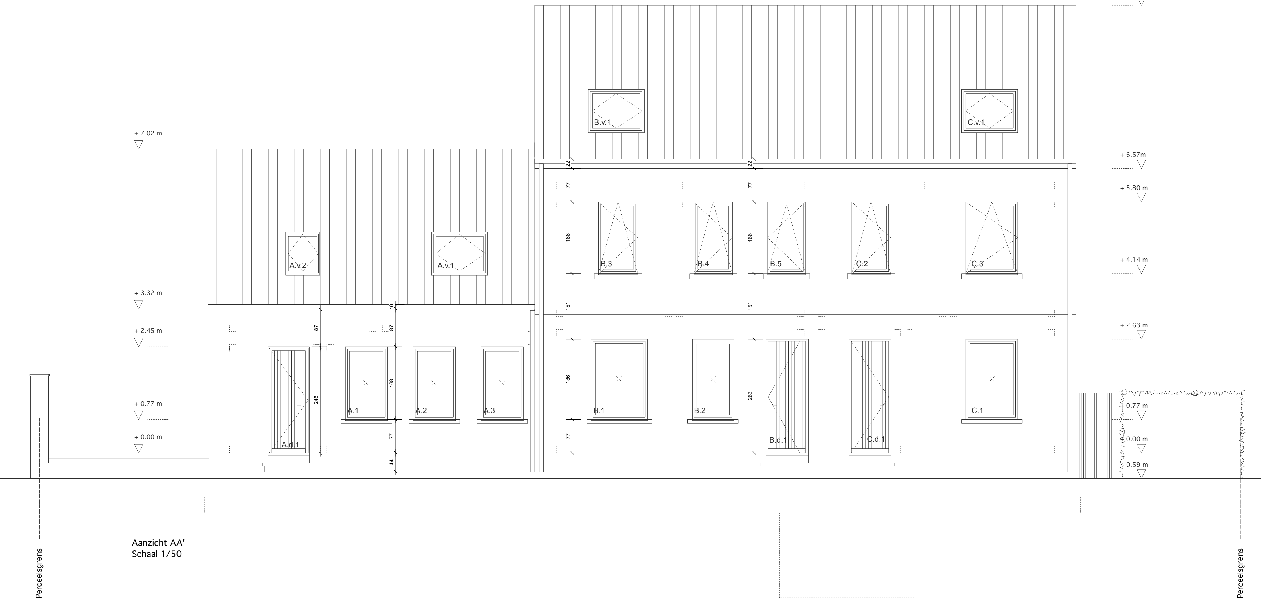
Aanzicht FF' Schaal 1/50
