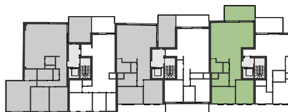
Grondplan niv. 3
