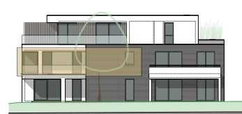
zuidgevel
