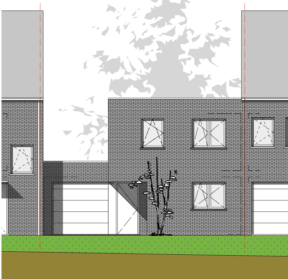
A2 VOORGEVEL
