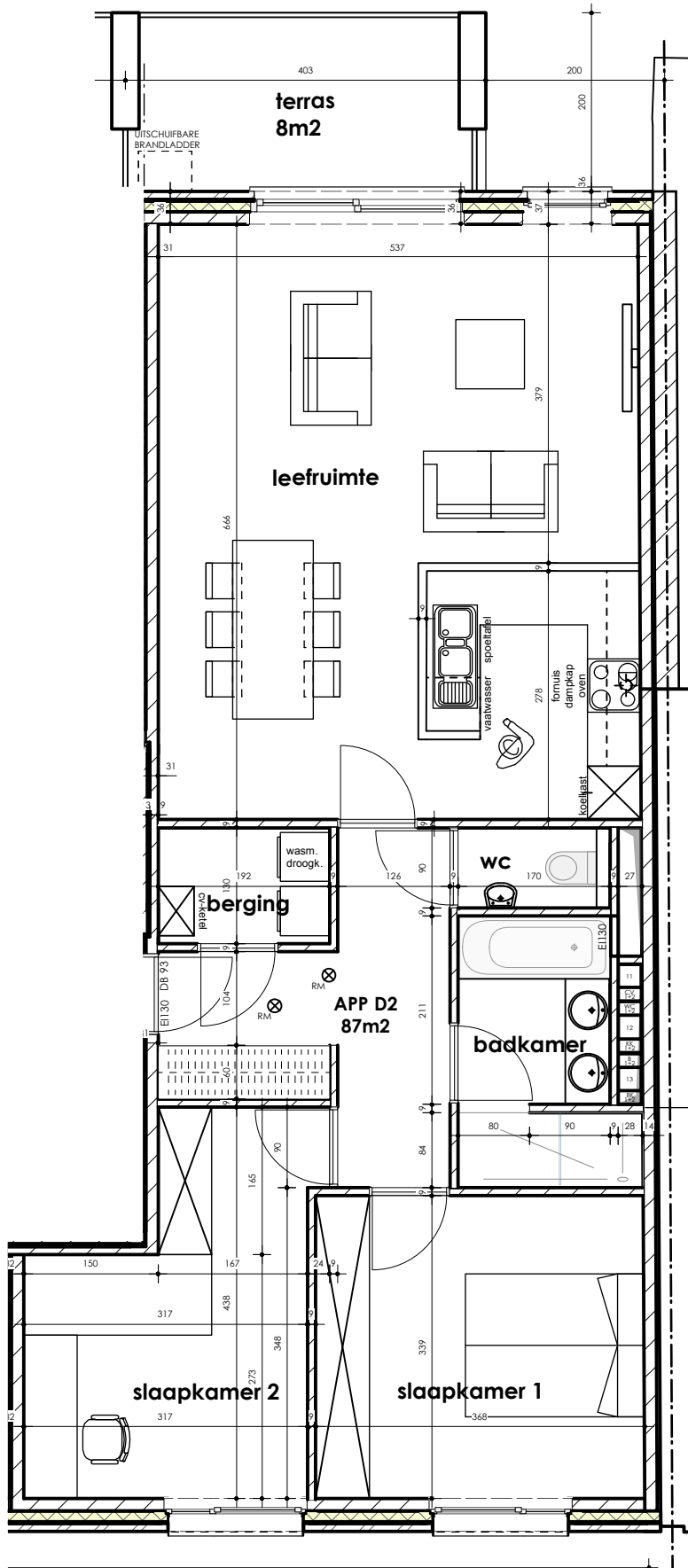
GRONDPLAN D2 1/75
