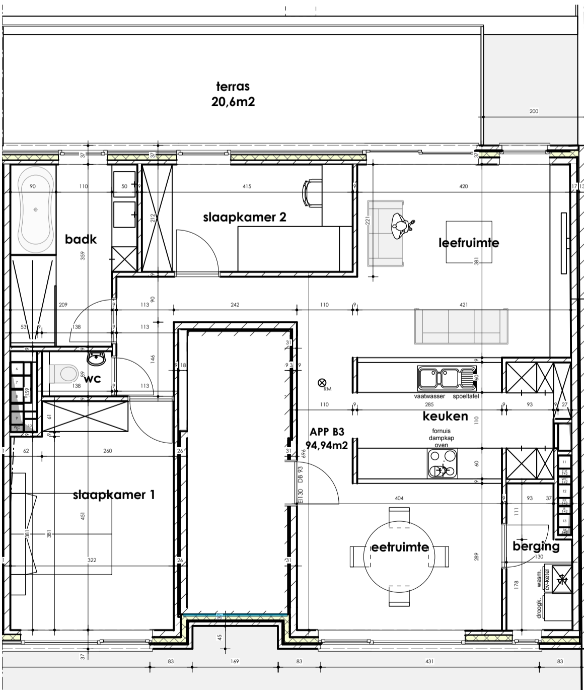
GRONDPLAN B3 1/75
