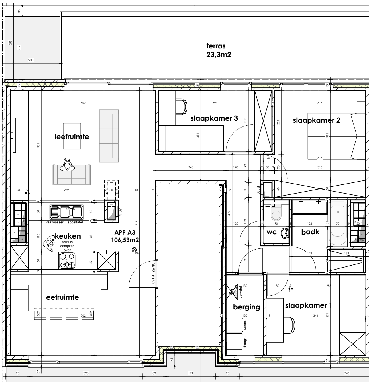
GRONDPLAN A3 1/75
