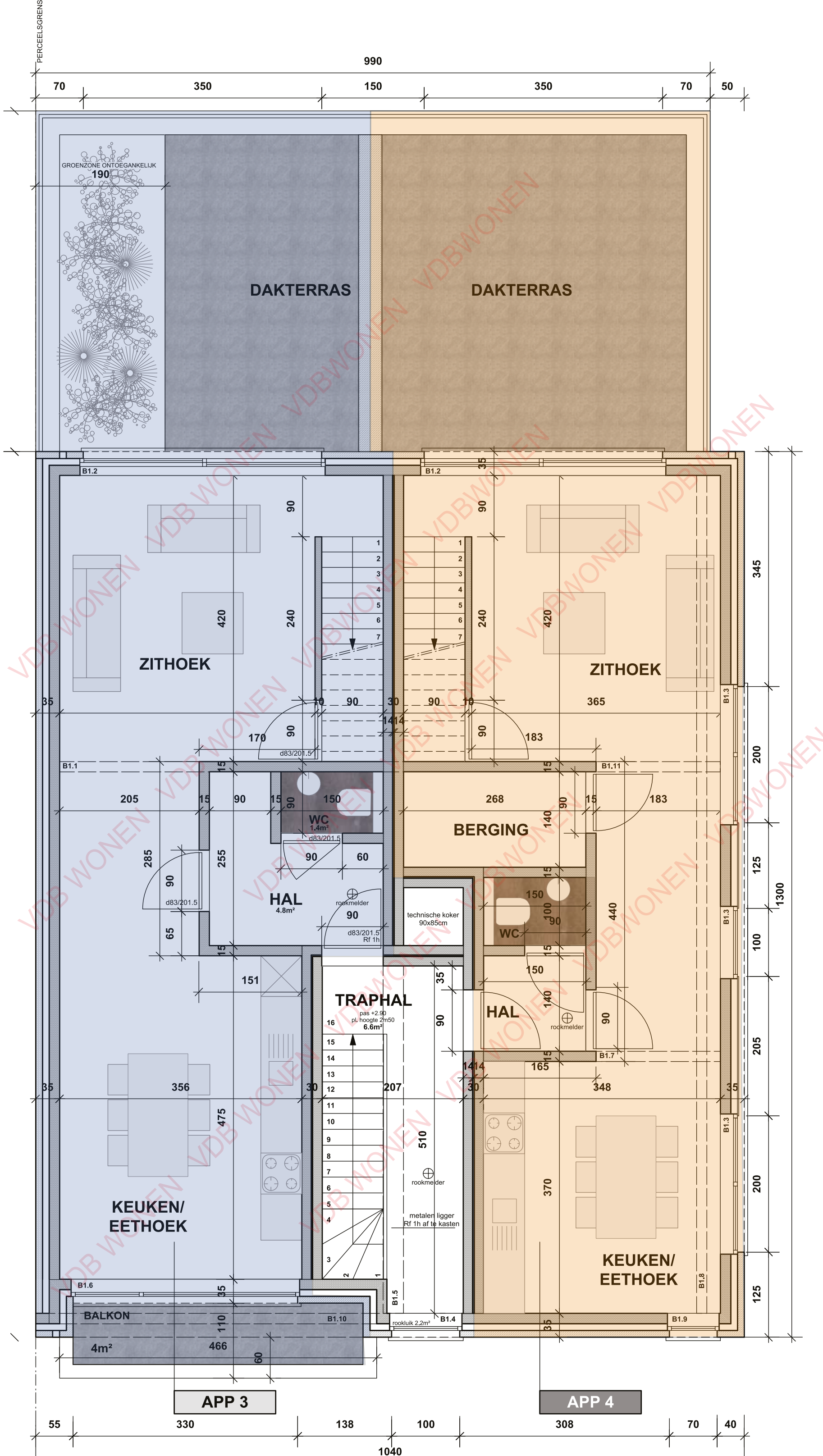
1° VERDIEPINGPLAN (app.3&4)
